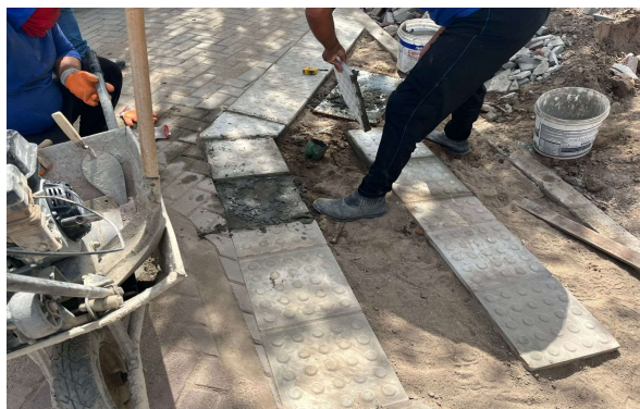
FOTO 3: PISO PODOTÁTIL
