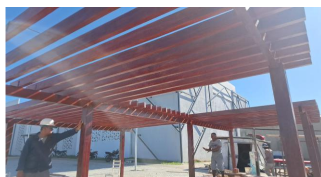
FOTO 14: CONFEÇÃO E INSTALAÇÃO DO PERGOLADO DE MADEIRA
